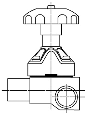
CCB-Ventil mit Handrad Vanne type CCB avec volant
