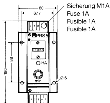
Bild 2: Einbaumaße Steuerautomat PRS 5-c, Tiefe 214
