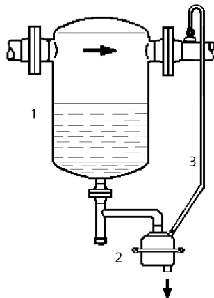
2 condensate trap
